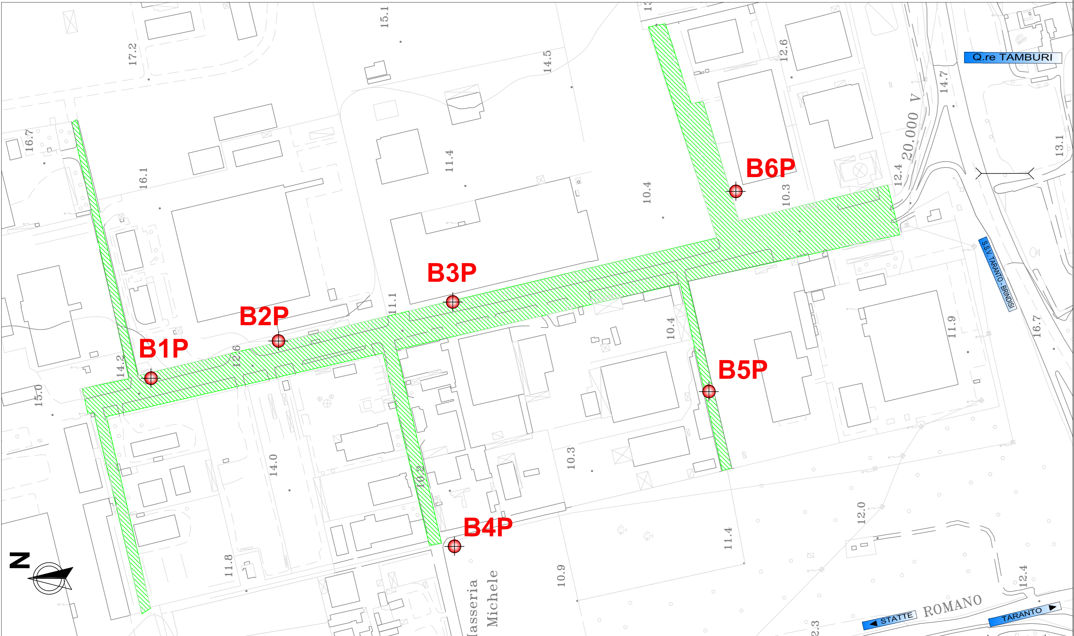
SONDAGGI CON PIEZOMETRO
